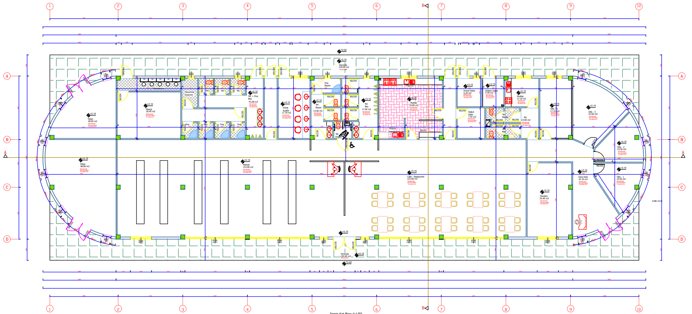
Zemin Kat Planı 0:1/50
